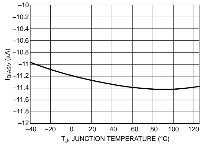
Figure 12. I_{BIASV} at V_{CC} = 15\text{ V} , V_{SNS} > V_{SNSBIAS}
